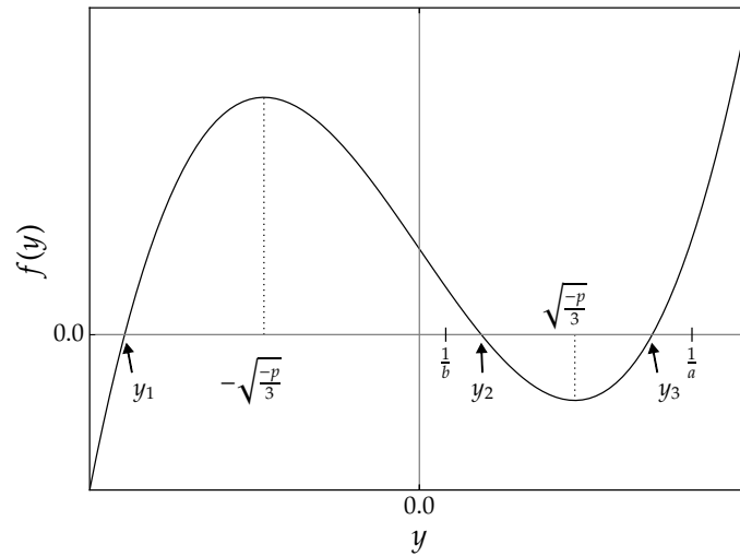
図 3: f(y) の概形
