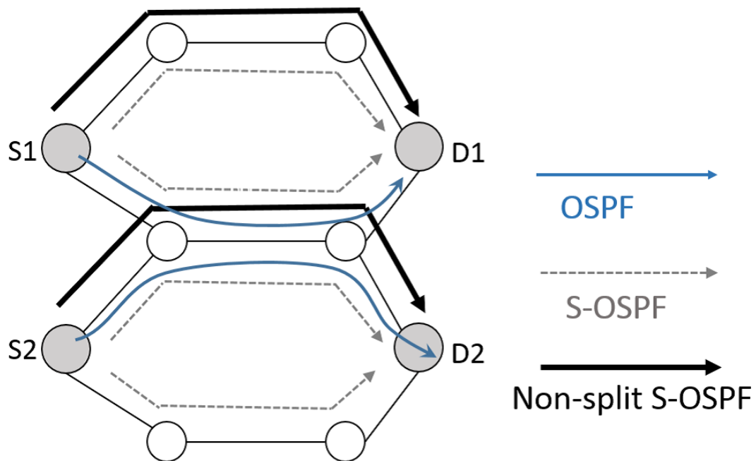
図 2.2: non-split S-OSPF と他のルーティング
