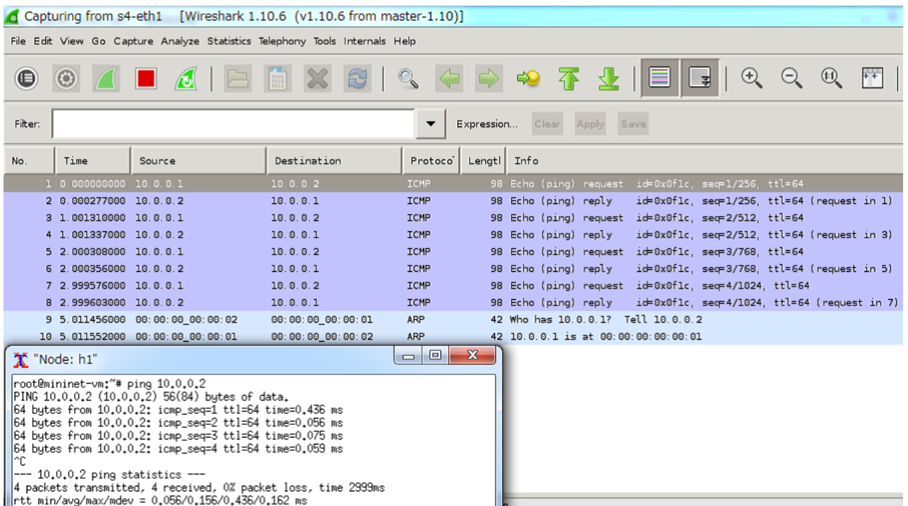
図 4.8: 経路変更後、h1 から h2 へ ping を打った際の s4-eth1 のパケットの動き
