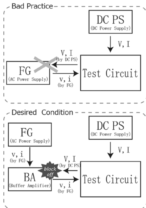
図 1. 測定機器の構成
