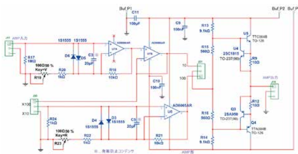
図8. アンプ部の回路構成
